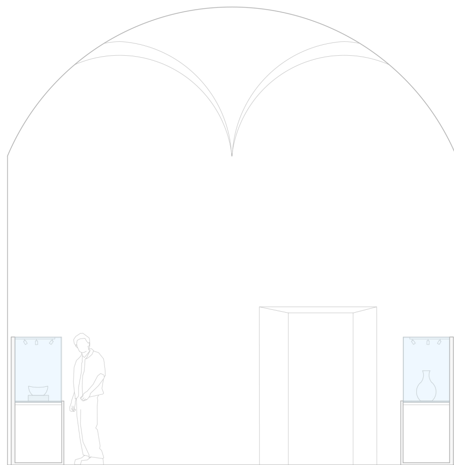
sezione BB'
